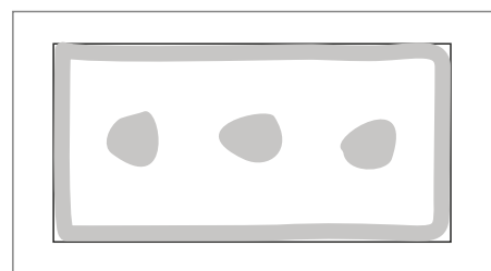
6. Applicazione del collante TECNOFIX P10 sul pannello
